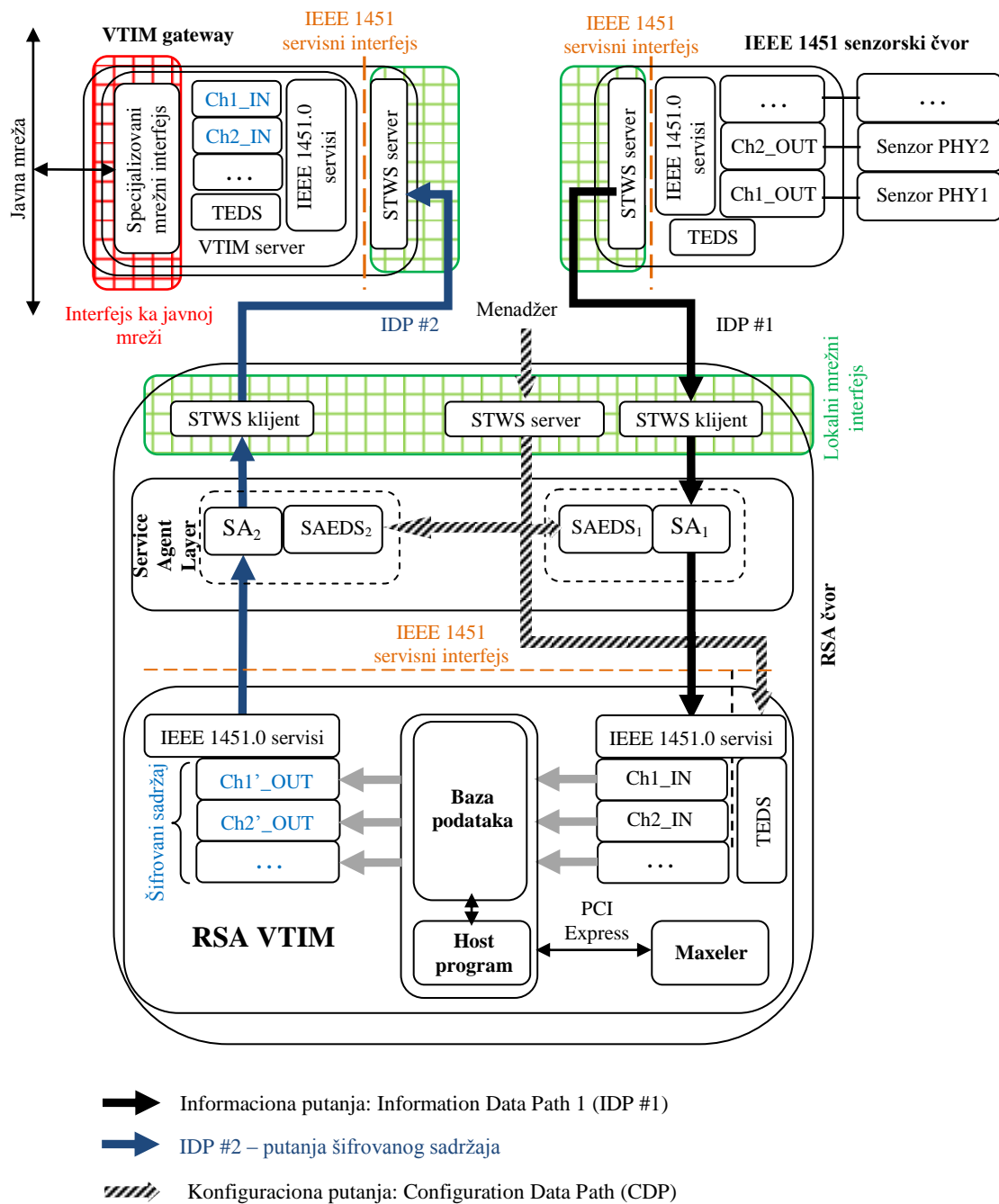
Slika 5.4 Koncept integracije Maxeler platforme u VTIM formi za potrebe ubrzanja procesa enkripcije podataka u lokalnoj servisno orijentisanoj mreži pametnih pretvarača.
